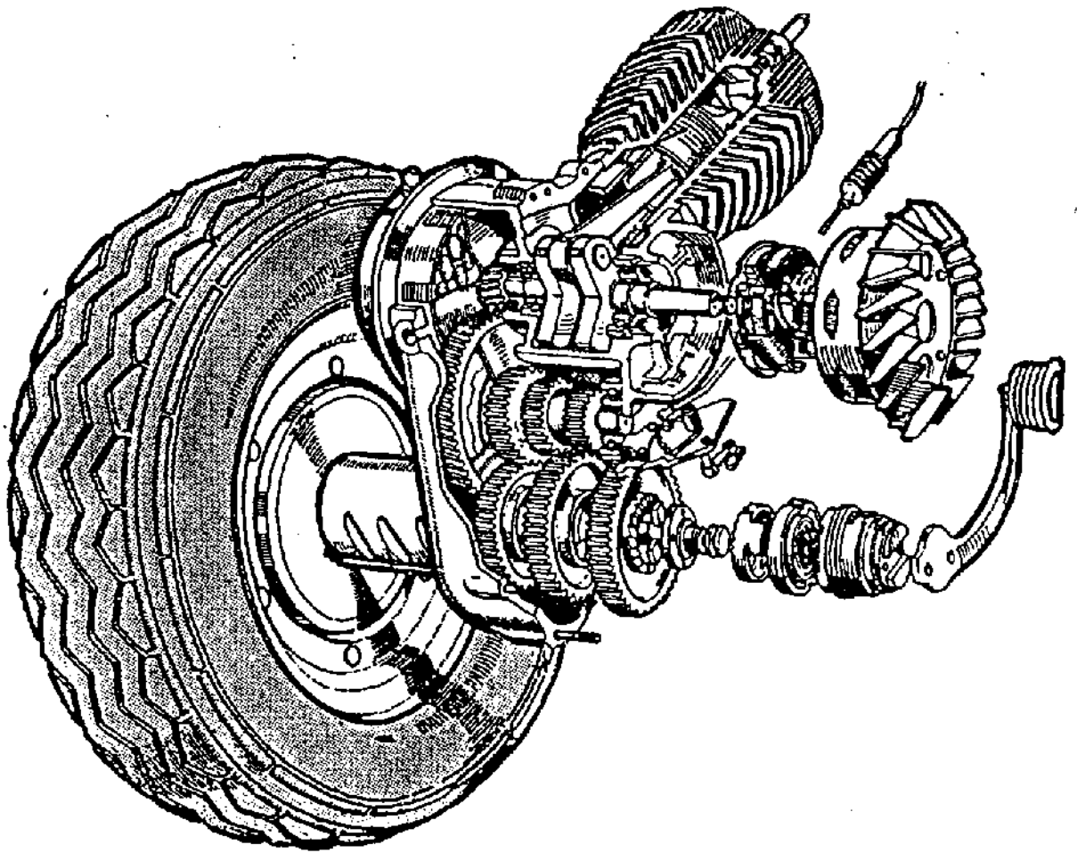
Conjunto del bloque motor y rueda trasera.
