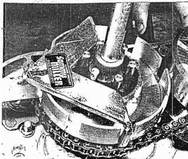
Foto 35 Bloqueado del embrague para poder aflojar la tuerca de sujeción
