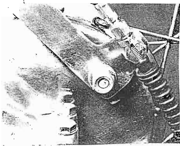
Foto 153 Apretar los tornillos del armazón del freno
