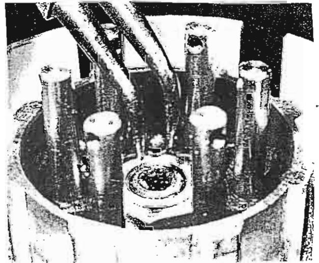
Foto 78 Sujetar la bola de presión con grasa
