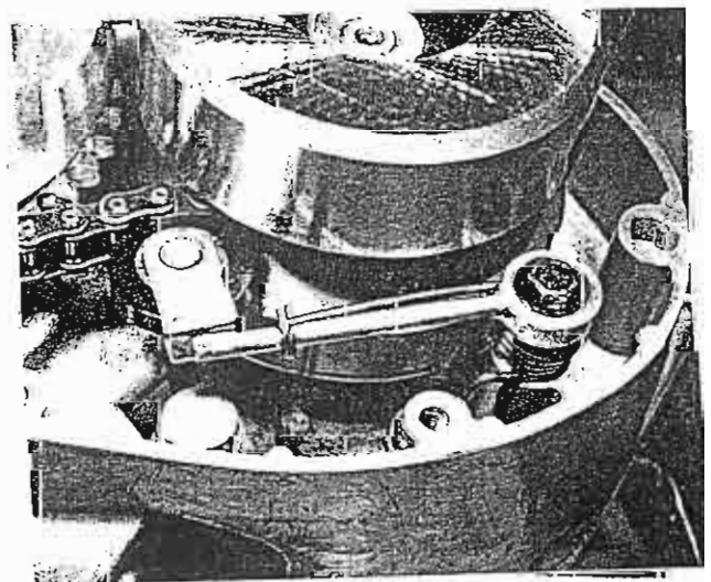
Foto 80 Colocación del tensor de la cadena primaria con el muelle
