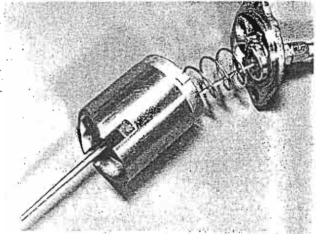
Foto 109 Antes de su montaje se comprobará el posible desgaste de la campana
