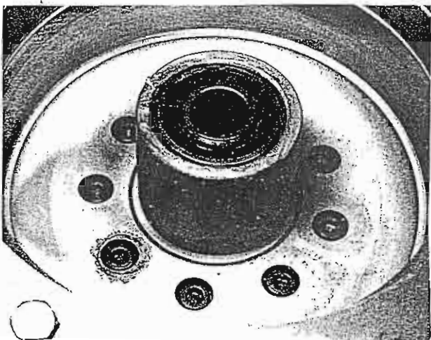
Foto 170 Hueve tornillos sujetan el tambor de freno trasero
