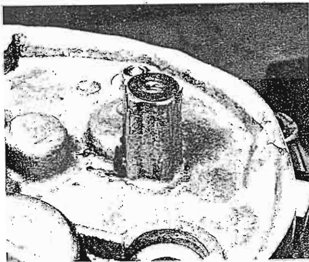
Foto 86 Antes de la colocación de la tapa, se sujetará la junta mediante grasa
