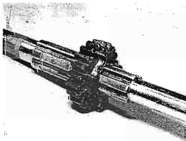
Foto 55 Sacar el piñón intermedio de la 3ª marcha
