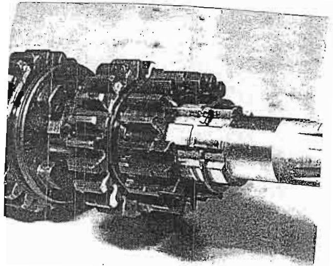
Foto 50 Desmontaje del aro de seguridad
