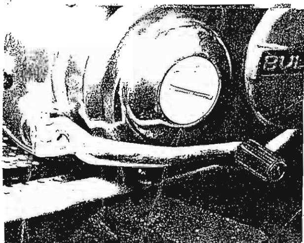
Foto 12 Tornillo sujetador de la palanca del cambio
