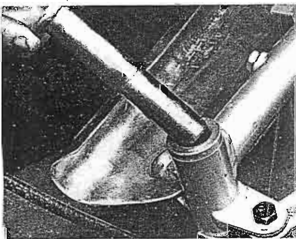
Foto 159 Desmontaje de los casquillos antifricción
