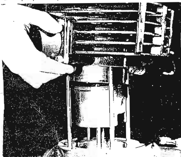
Foto 15 Sujetar el pistón al levantar el cilindro
