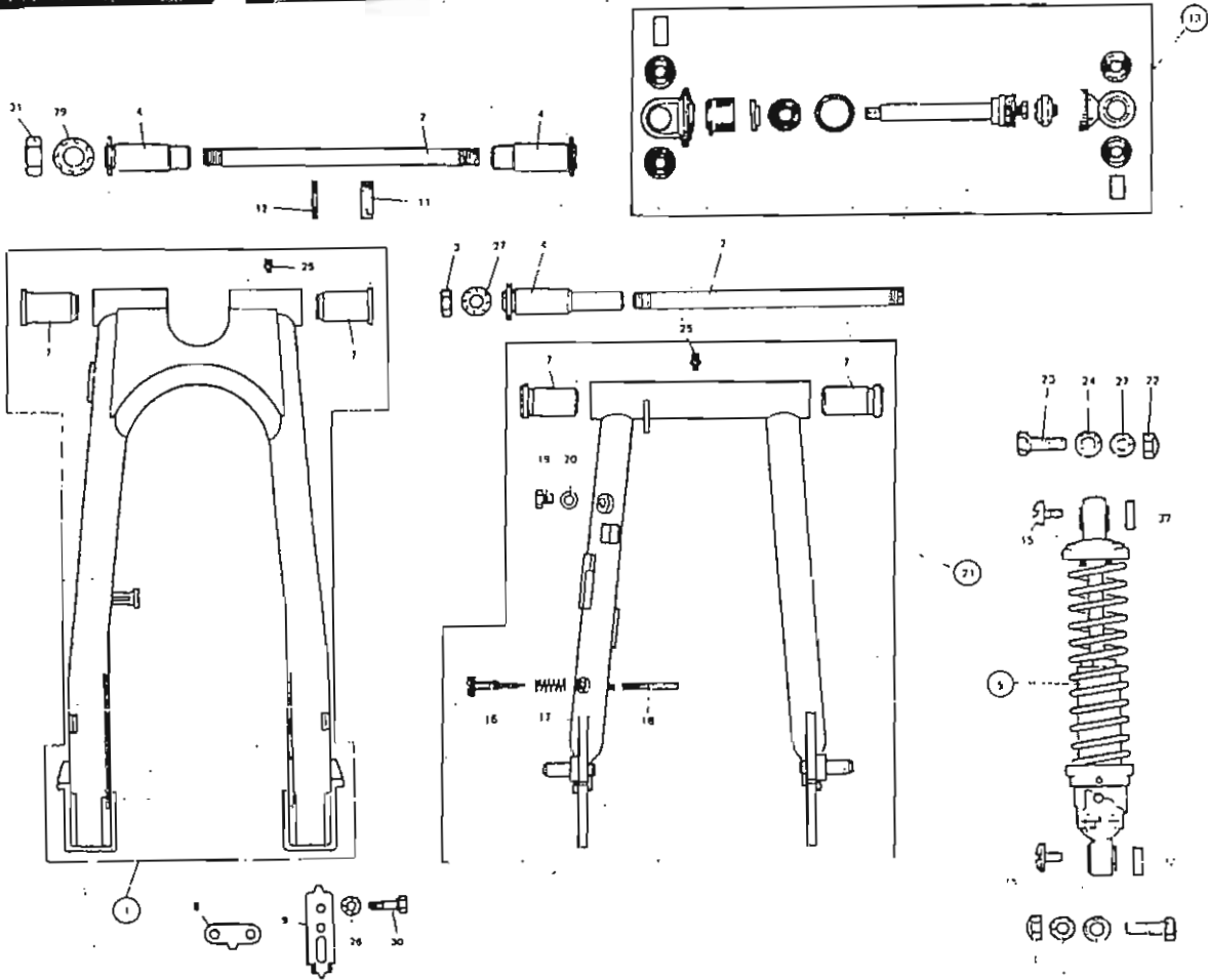
Grabado 164 Conjunto completo del basculante
