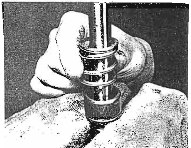
Foto 147 Embolo del amortiguador y muelle
