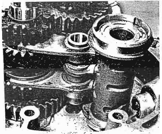
Foto 68 Introducir el rodillo y las horquillas del cambio en la caja
