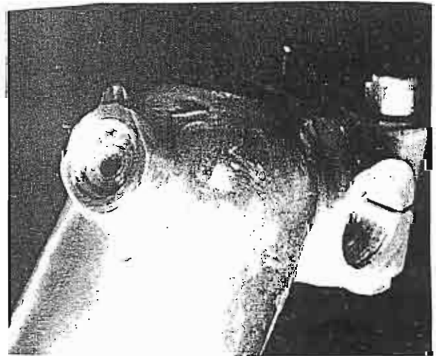
Foto 141 Salida del aceite del amortiguador
